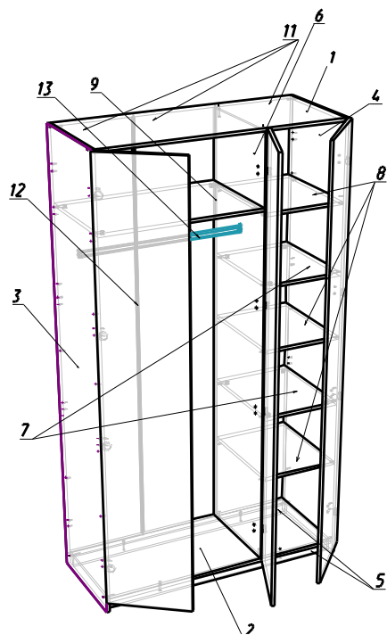
Рис.1 Схема сборки
